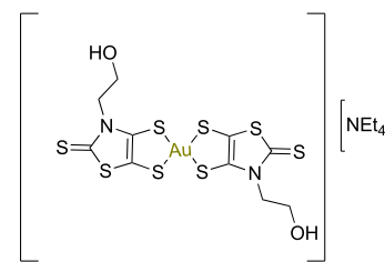
Au(III)-dithiolate-4
